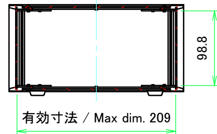
A-A ( 1 : 5 )
