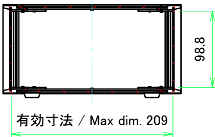
A-A ( 1 : 5 )
