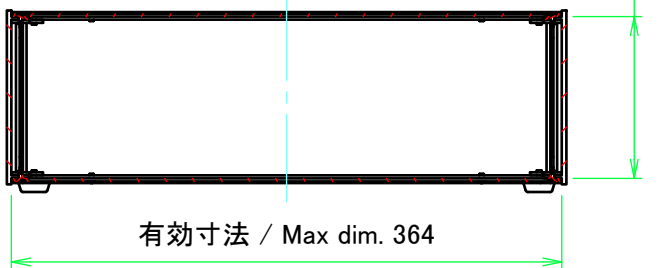
C-C ( 1 : 5 )
