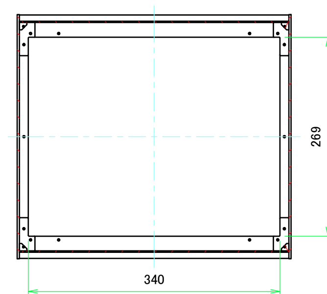
B-B ( 1 : 5 )
