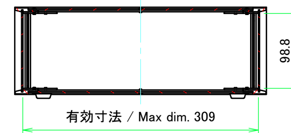
A-A ( 1 : 5 )
