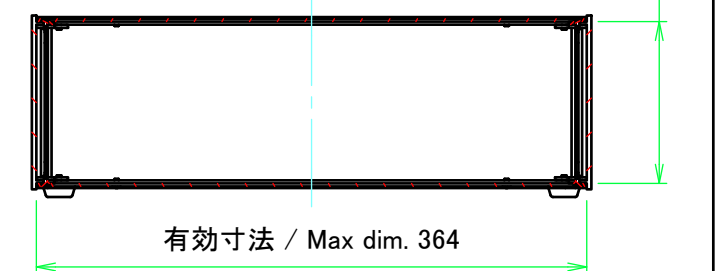
C-C ( 1 : 5 )
