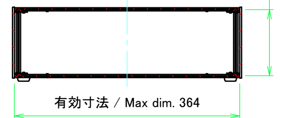
C-C ( 1 : 6 )
