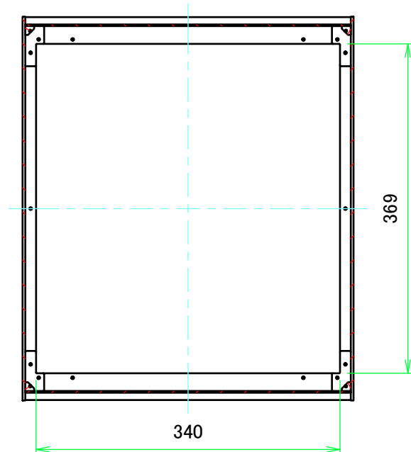
B-B ( 1 : 6 )
