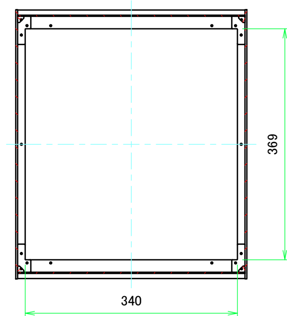
B-B ( 1 : 6 )
