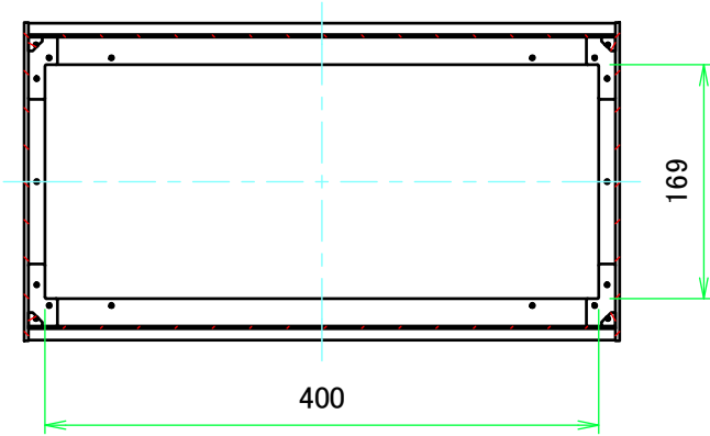
B-B ( 1 : 6 )
