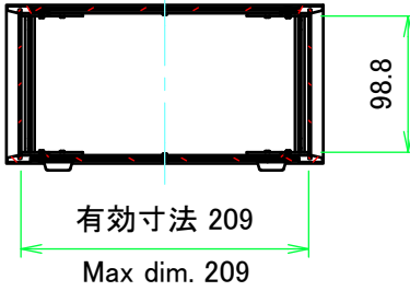
A-A ( 1 : 6 )
