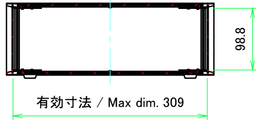
A-A ( 1 : 6 )
