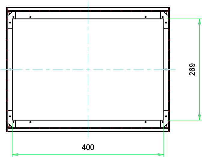
B-B ( 1 : 6 )
