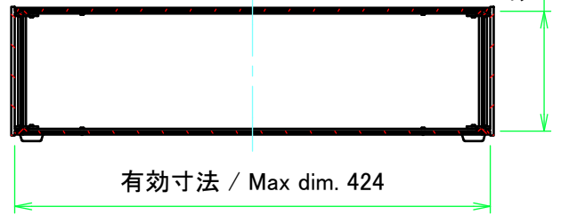
C-C ( 1 : 6 )
