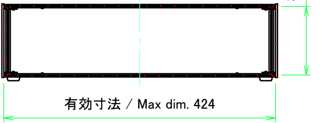
C-C ( 1 : 6 )
