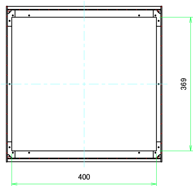
B-B ( 1 : 6 )
