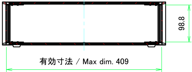
A-A ( 1 : 6 )
