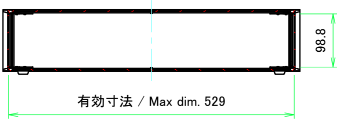
A-A ( 1 : 7 )
