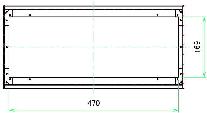
B-B ( 1 : 6 )
