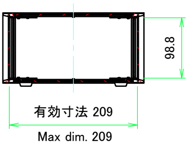
A-A ( 1 : 6 )
