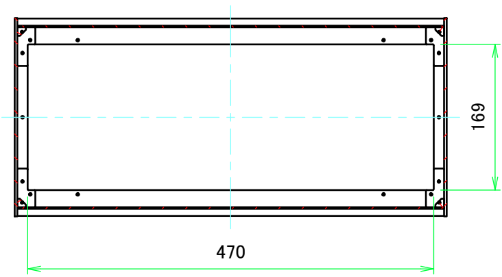
B-B ( 1 : 6 )
