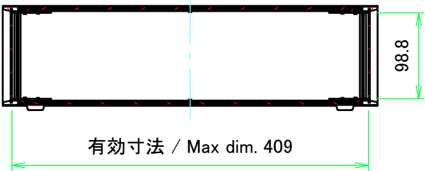
A-A ( 1 : 6 )
