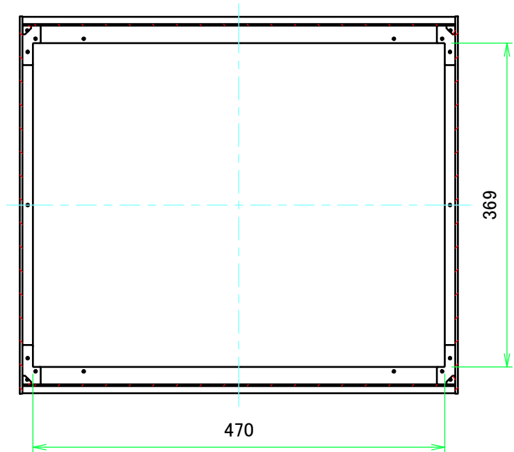
B-B ( 1 : 6 )
