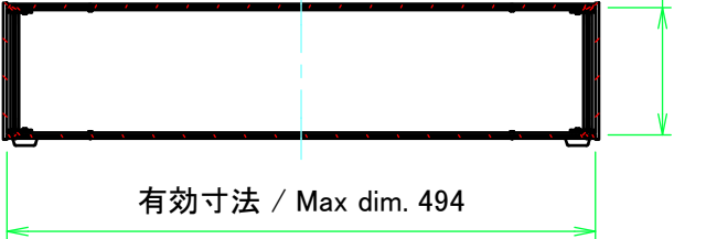
C-C ( 1 : 7 )
