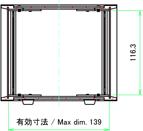
A-A (1:3)
