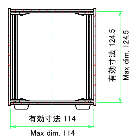
C-C ( 1 : 3 )
