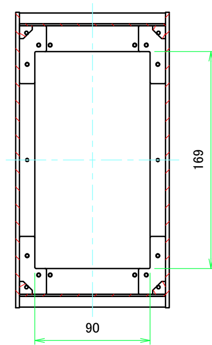
B-B ( 1 : 3 )
