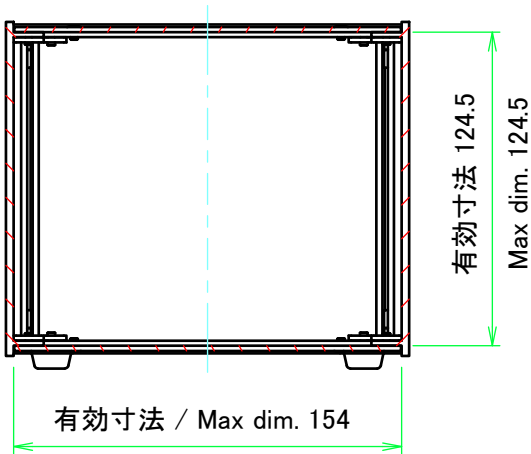
C-C ( 1 : 3 )
