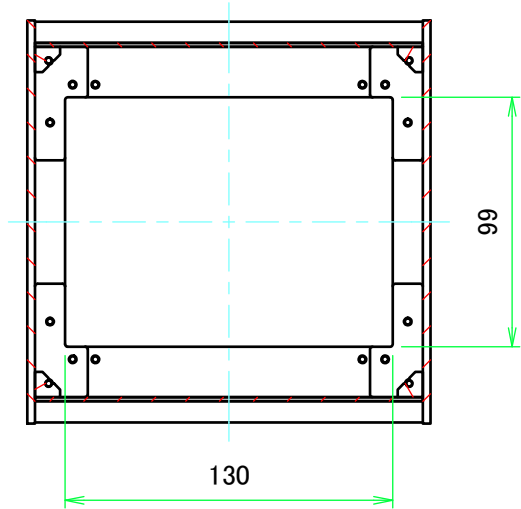
B-B ( 1 : 3 )
