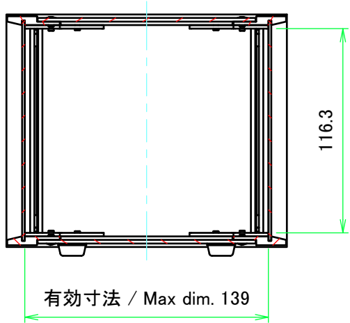
A-A ( 1 : 3 )
