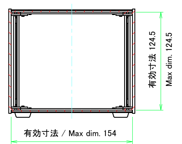
C-C ( 1 : 3 )
