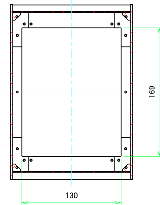
B-B ( 1 : 3 )
