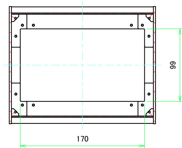
B-B ( 1 : 3 )
