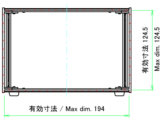
C-C ( 1 : 3 )
