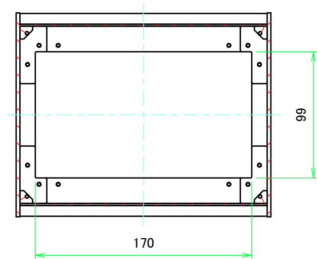
B-B ( 1 : 3 )
