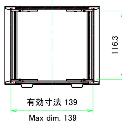
A-A ( 1 : 4 )
