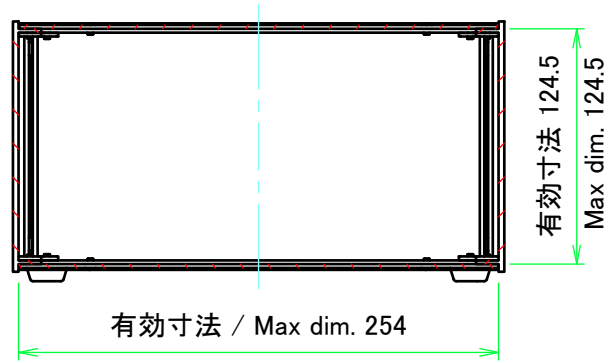
C-C ( 1 : 4 )
