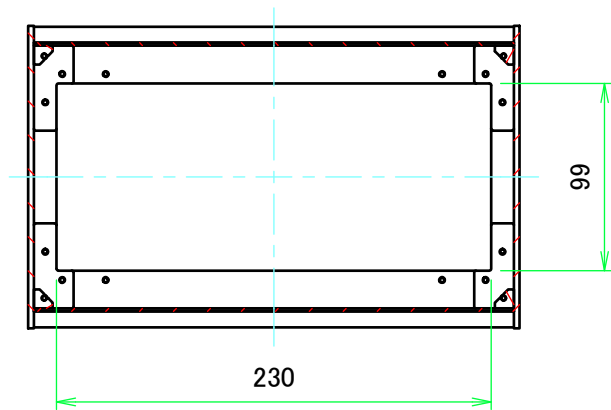
B-B ( 1 : 4 )
