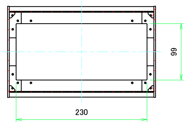
B-B ( 1 : 4 )
