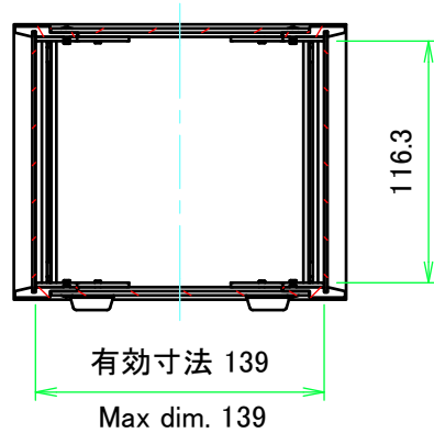
A-A ( 1 : 4 )
