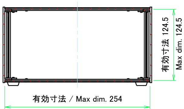
C-C ( 1 : 4 )
