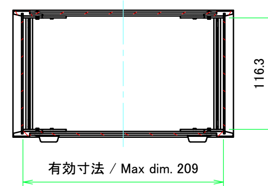
A-A ( 1 : 4 )
