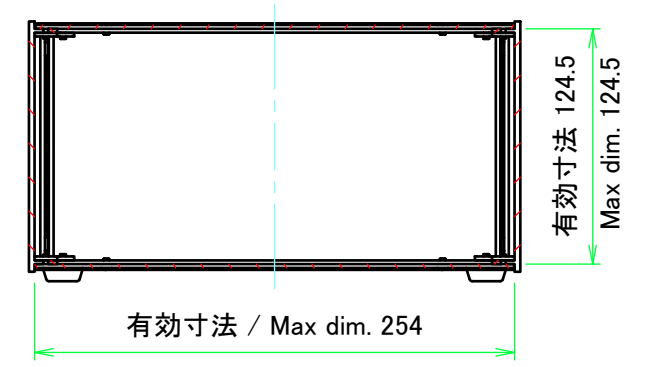
C-C ( 1 : 4 )
