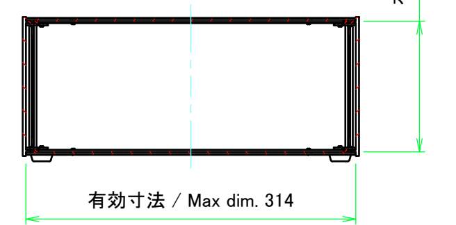
C-C ( 1 : 5 )
