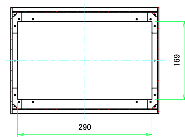
B-B ( 1 : 5 )
