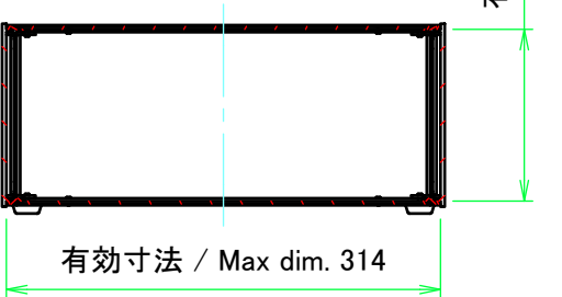
C-C ( 1 : 6 )
