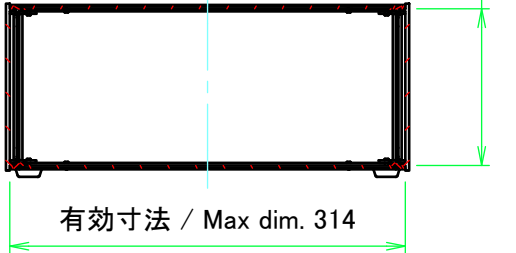
C-C ( 1 : 6 )
