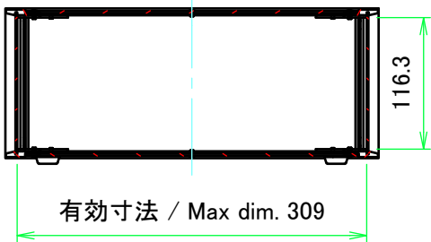
A-A ( 1 : 6 )
