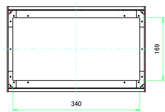
B-B ( 1 : 5 )
