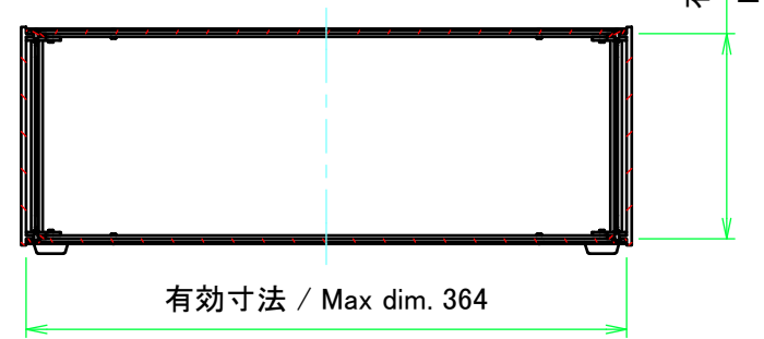
C-C ( 1 : 5 )
