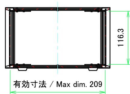
A-A ( 1 : 5 )
