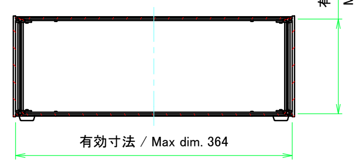
C-C ( 1 : 5 )
