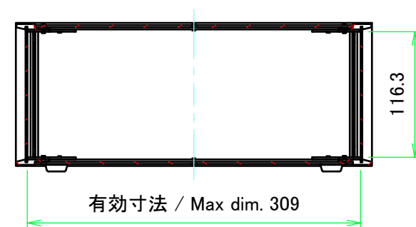
A-A ( 1 : 5 )
