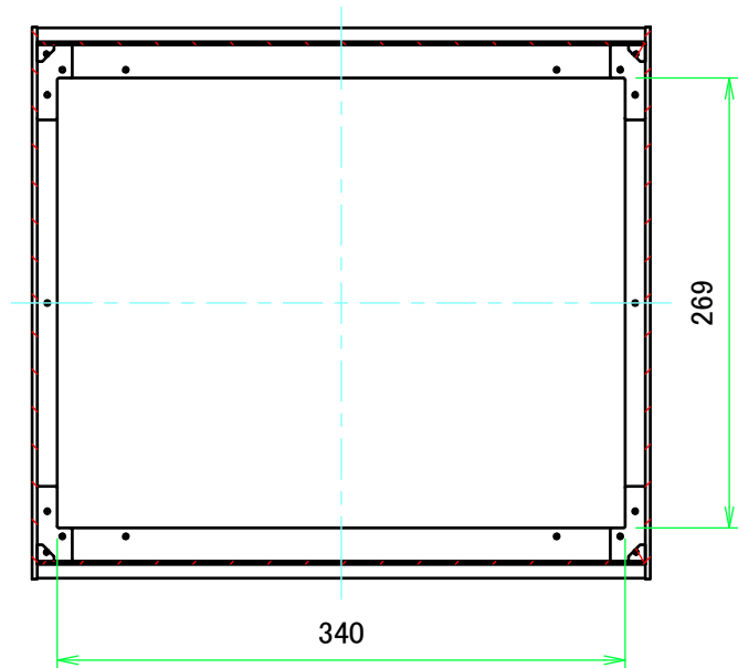
B-B ( 1 : 5 )
