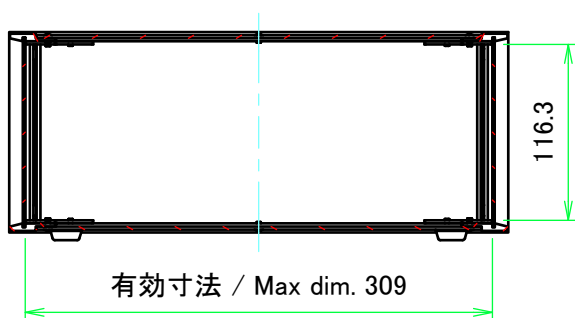
A-A ( 1 : 5 )
