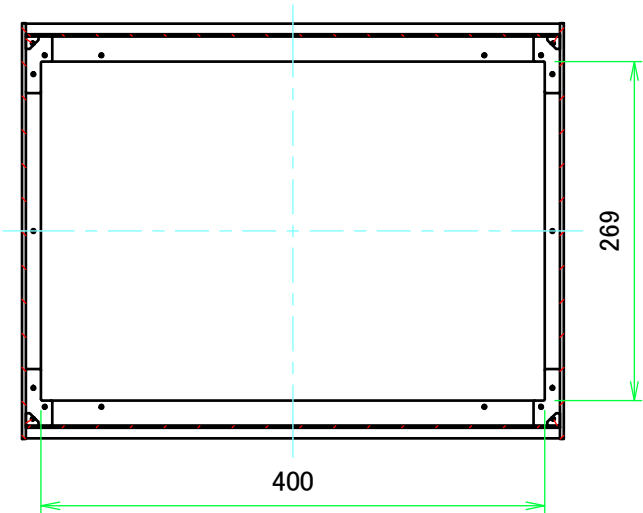
B-B ( 1 : 6 )
