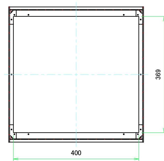
B-B ( 1 : 6 )
