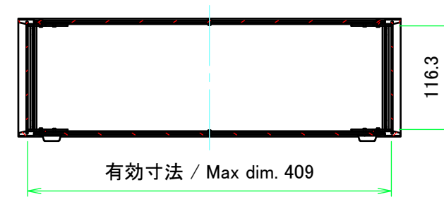
A-A ( 1 : 6 )
