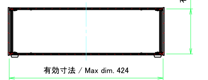
C-C ( 1 : 6 )
