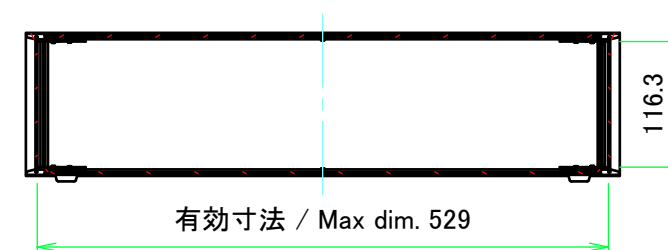
A-A (1:7)
