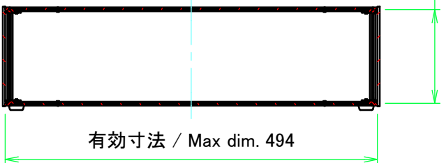
C-C ( 1 : 7 )
