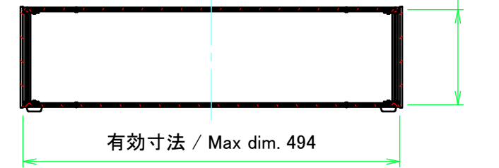
C-C ( 1 : 7 )
