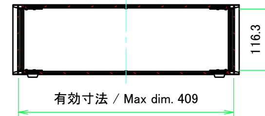
A-A ( 1 : 7 )
