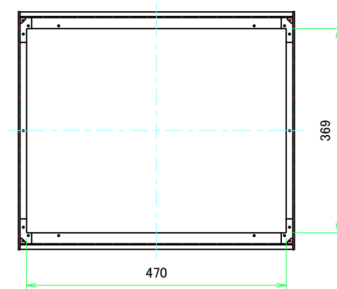
B-B ( 1 : 7 )
