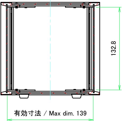
A-A (1:3)
