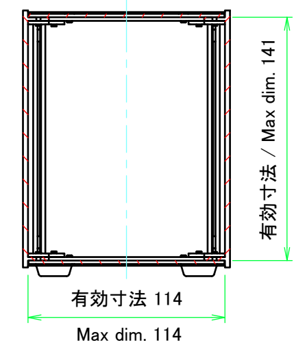
C-C ( 1 : 3 )
