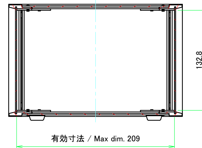
A-A ( 1 : 3 )
