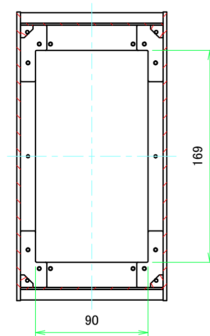
B-B ( 1 : 3 )
