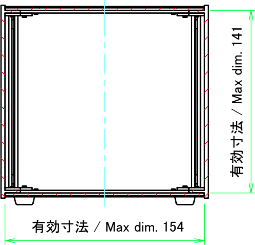
C-C ( 1 : 3 )
