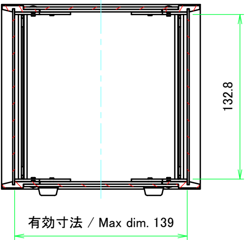
A-A ( 1 : 3 )
