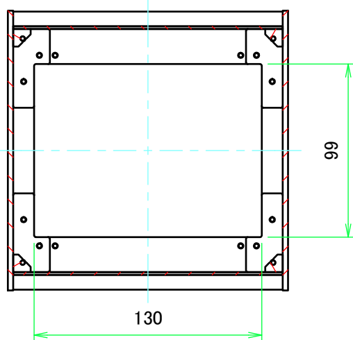
B-B ( 1 : 3 )
