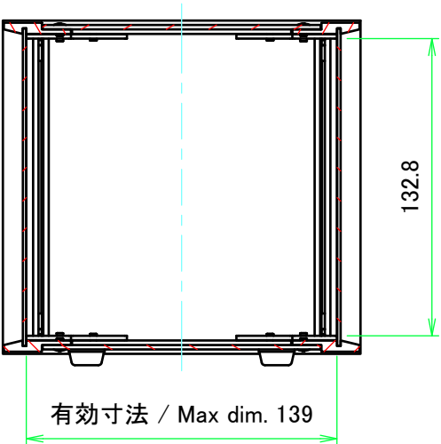
A-A ( 1 : 3 )
