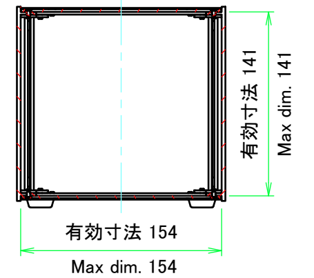
C-C ( 1 : 4 )
