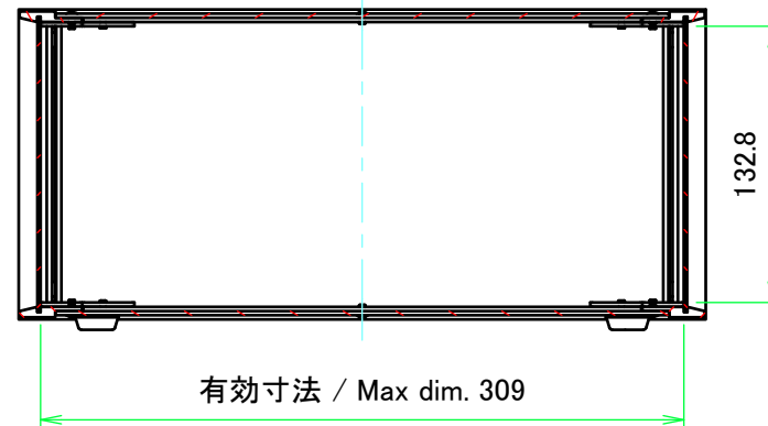
A-A ( 1 : 4 )
