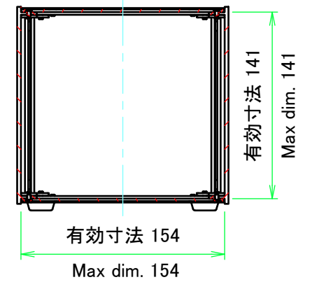
C-C ( 1 : 4 )
