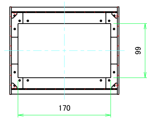
B-B ( 1 : 4 )
