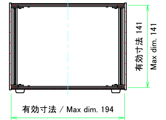
C-C ( 1 : 4 )
