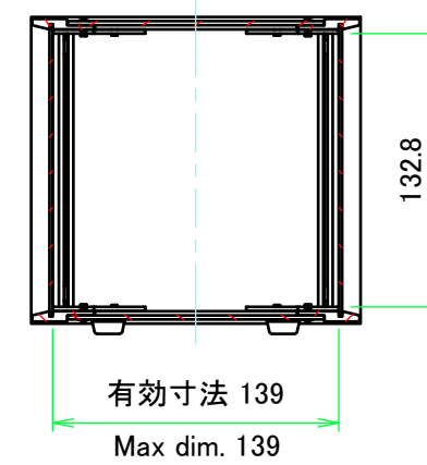
A-A ( 1 : 4 )
