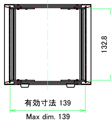
A-A ( 1 : 4 )
