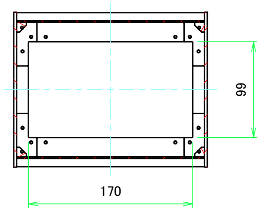
B-B ( 1 : 4 )
