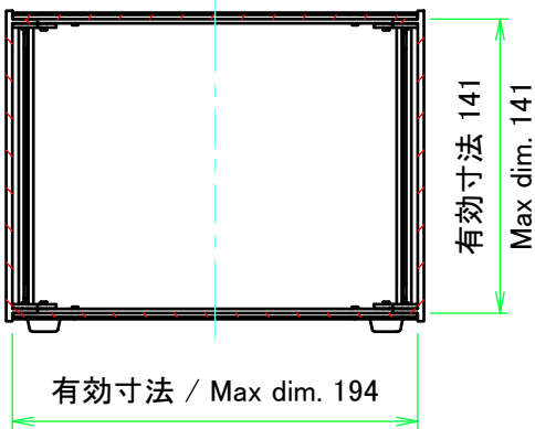
C-C ( 1 : 4 )
