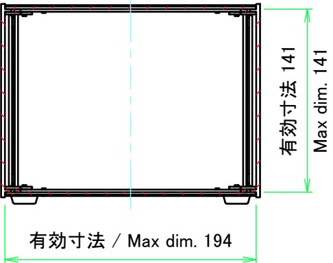
C-C ( 1 : 4 )
