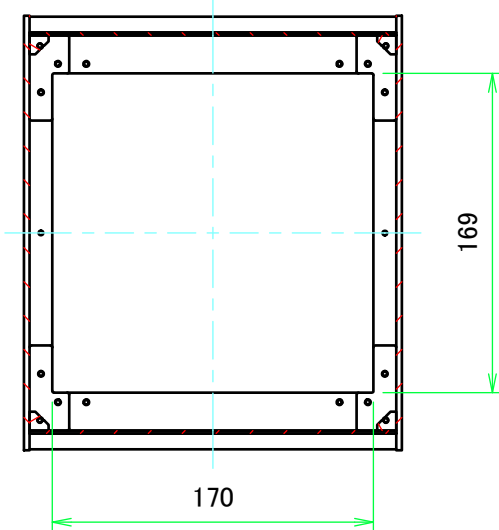
B-B ( 1 : 4 )
