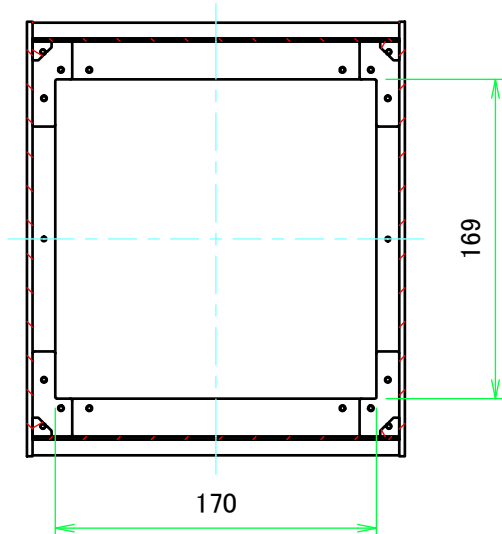
B-B ( 1 : 4 )
