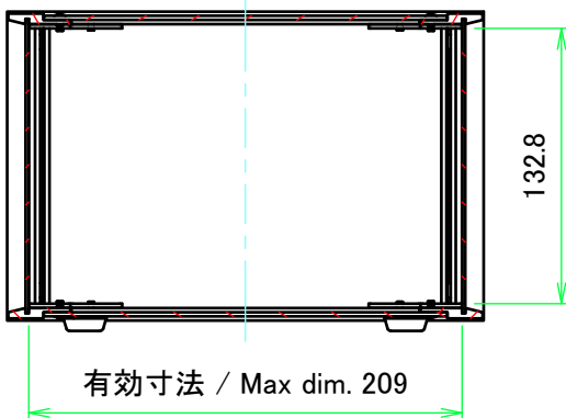
A-A ( 1 : 4 )
