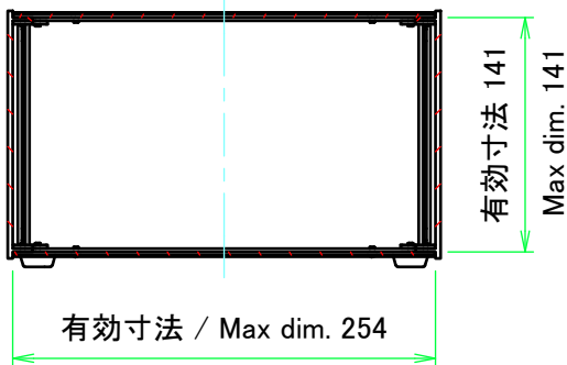
C-C ( 1 : 5 )
