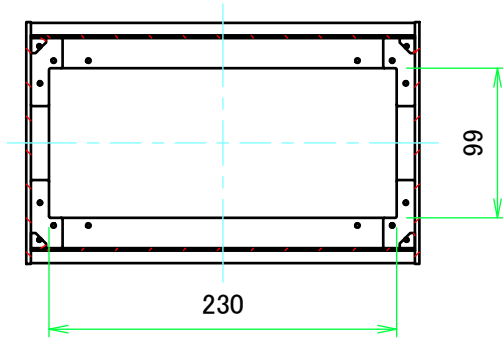
B-B ( 1 : 5 )
