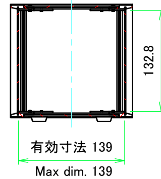
A-A ( 1 : 5 )
