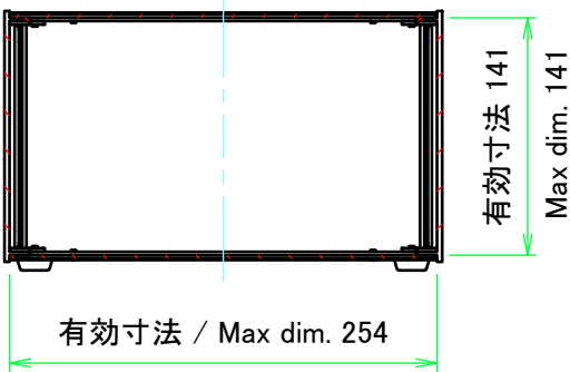
C-C ( 1 : 5 )
