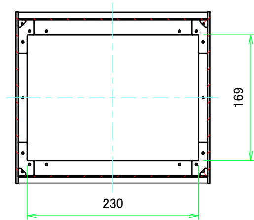
B-B ( 1 : 5 )
