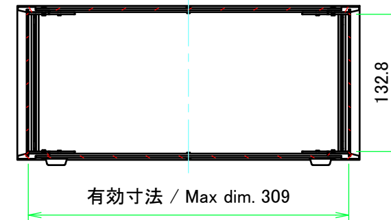
A-A (1:5)
