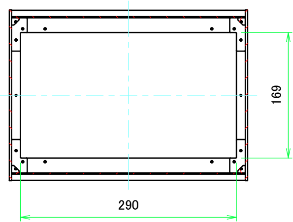
B-B ( 1 : 5 )
