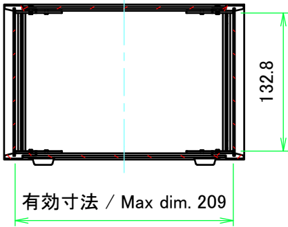
A-A ( 1 : 5 )
